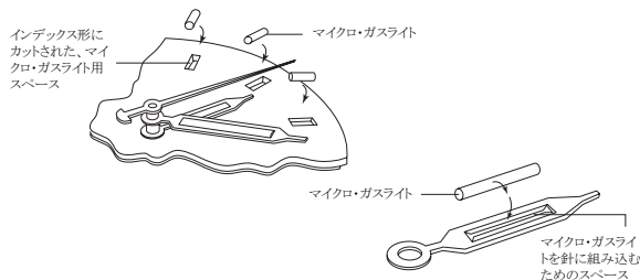
文字盤や針に組み込まれるマイクロ・ガスライト
