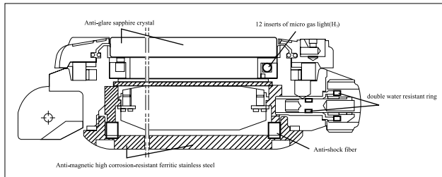
Schematische Ansicht eines antimagnetischen Gehäuses einer BALL-Uhr
