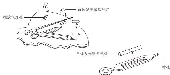
自体发光微型气灯装嵌图
