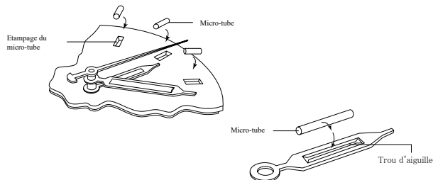
Diagramme représentant la fixation des micro-tubes sur les aiguilles et le cadran
